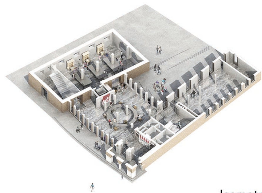
Isometrie EG
