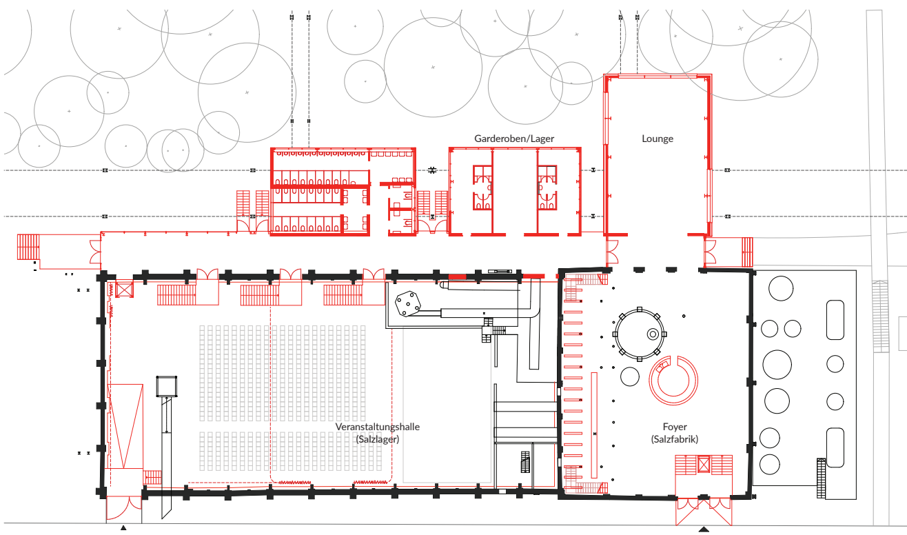
Grundriss Salzlager mit Erweiterungsbau
