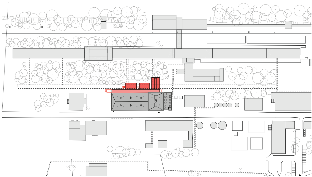
Lageplan Salzlager im Ensemble der Kokerei Hansa
