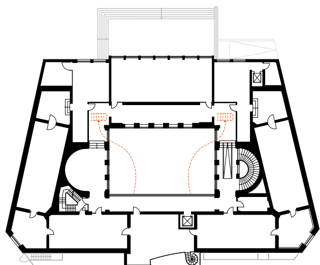
Entrauchung
