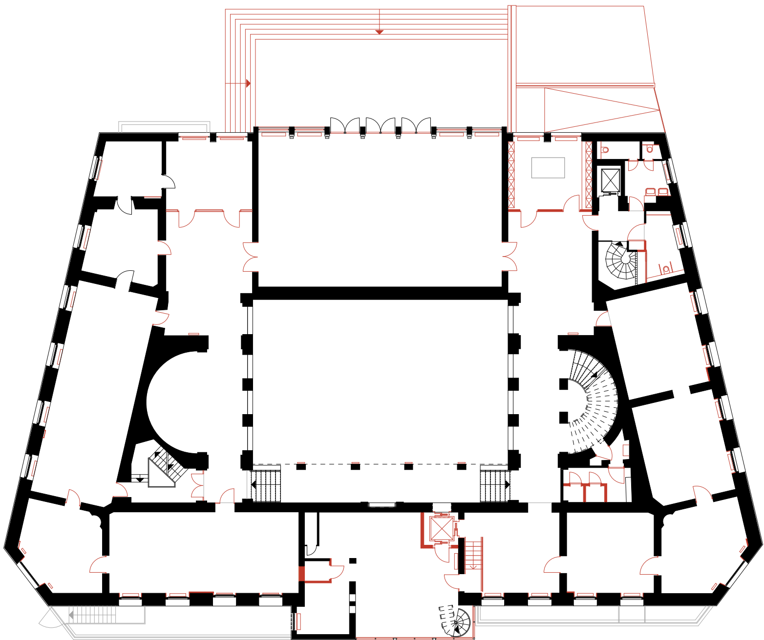
Grundriss EG
