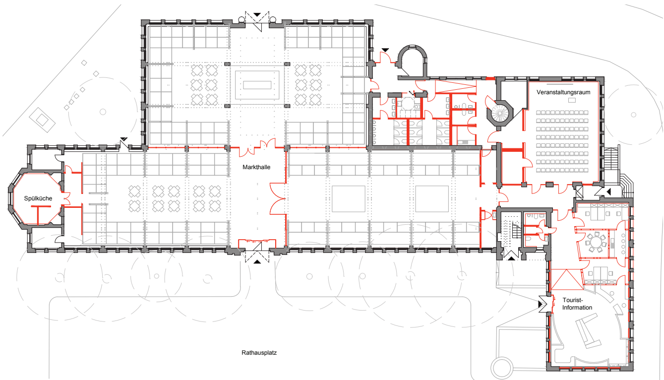
Grundriss
