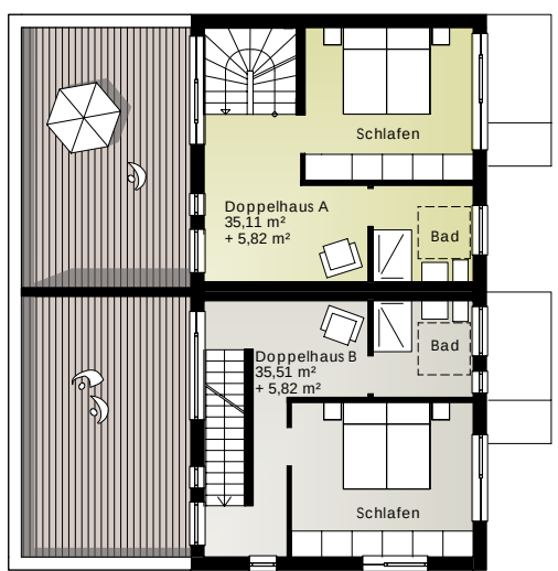
Grundriss 2.OG – Reihenhaus M1:150
