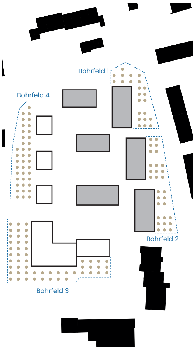
Energie Konzeptpikto – Tiefenbohrfelder
