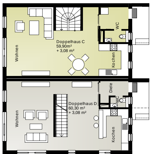
Grundriss EG – Reihenhaus M1:150
