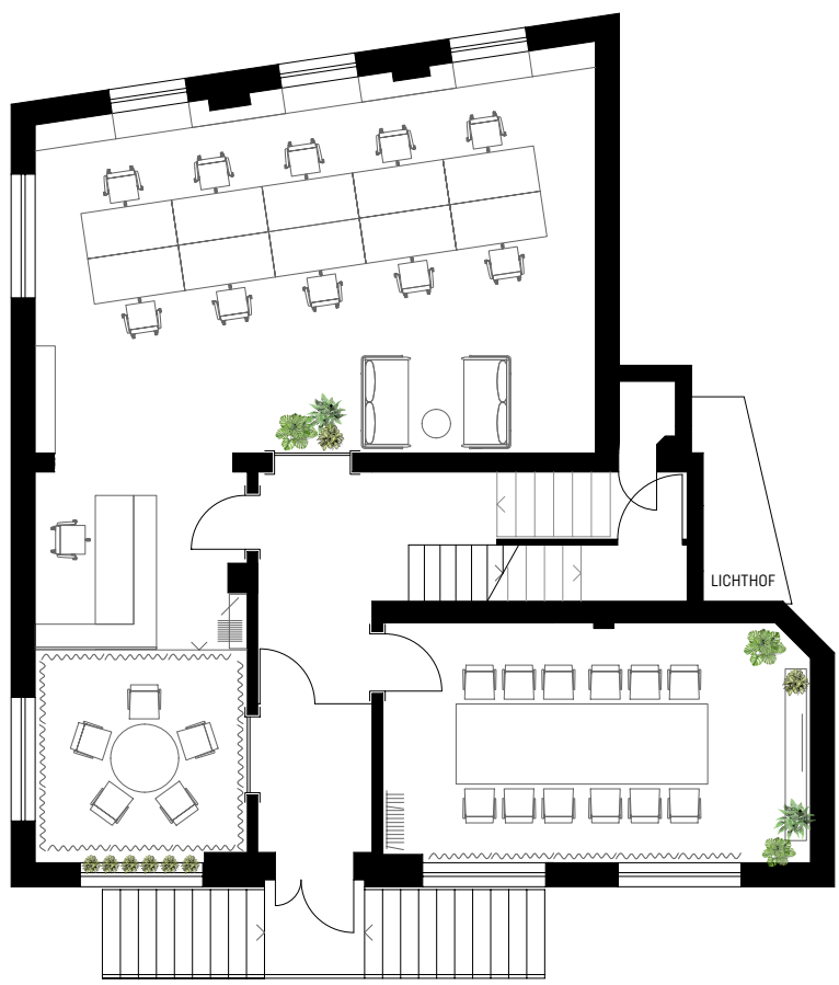
Erdgeschoss o.M.
